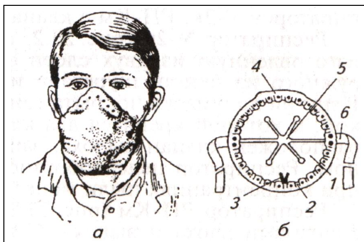
Рисунок – 2.1 – Респиратор типа «Лепесток»: а – общий вид; б – устройство; 1 – корпус; 2 – обтюратор; 3 – резиновый шнур; 4 – алюминиевая пластинка внутри обтюратора; 5 – пластмассовая распорка; 6 – завязки
