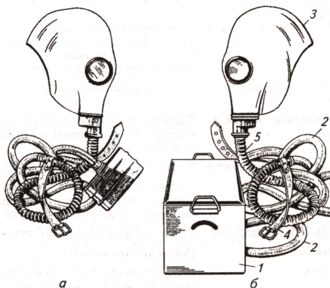
Рисунок 2.5 – Шланговые противогазы:
