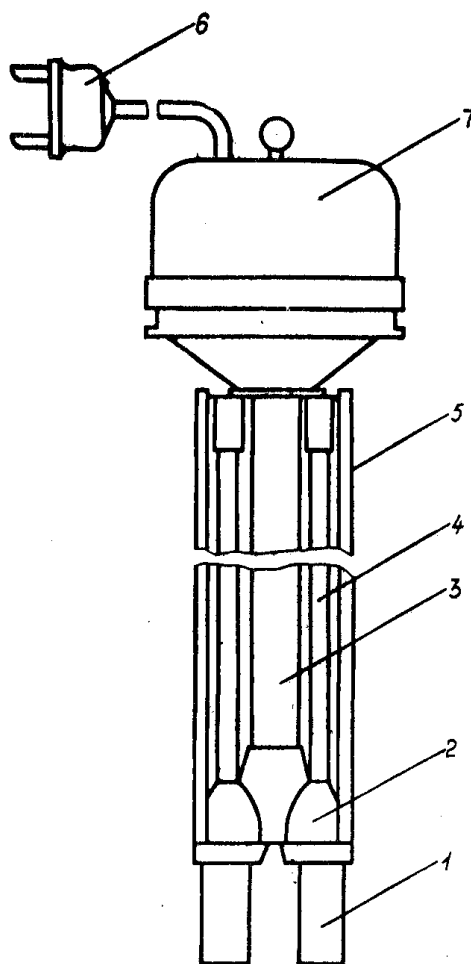
Рисунок 2.1 – Психрометр аспирационный М-34:
