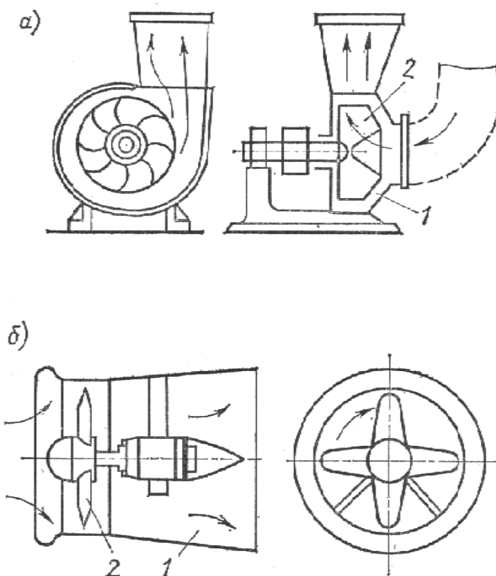
Рисунок 1.1 – Вентиляторы:
