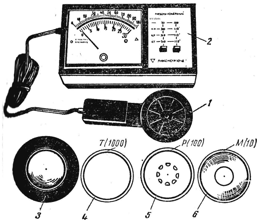
Рисунок 1.1 – Люксметр Ю-116:
