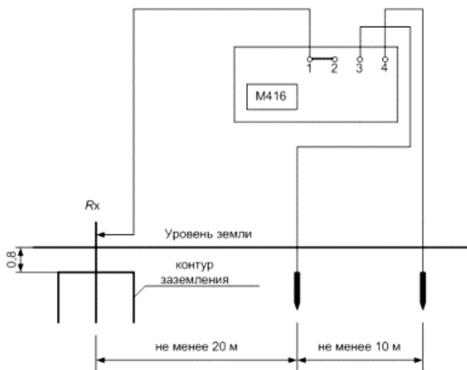
Рисунок 2.3 – Электрическая схема для измерения сопротивления заземляющего устройства
