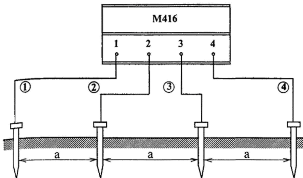
Рисунок 2.2 – Электрическая схема для определения удельного сопротивления грунта
