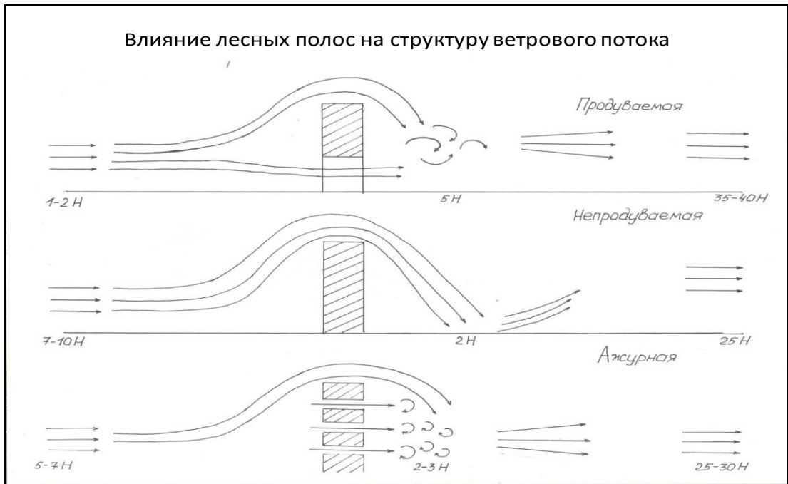
Рисунок 2.1 Влияние лесных полос различной конструкции на ветровой поток
