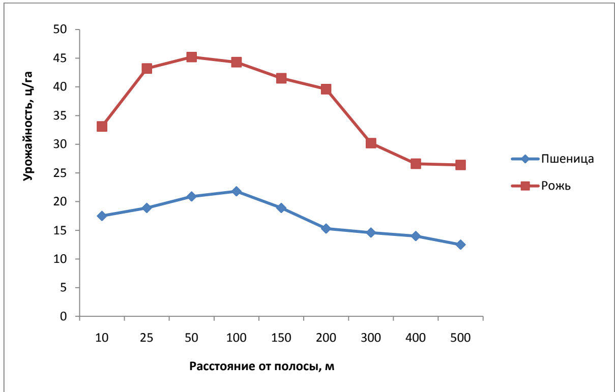
Рисунок 2.5 Влияние лесополосы продуваемой конструкции на урожайность сельскохозяйственных культур
