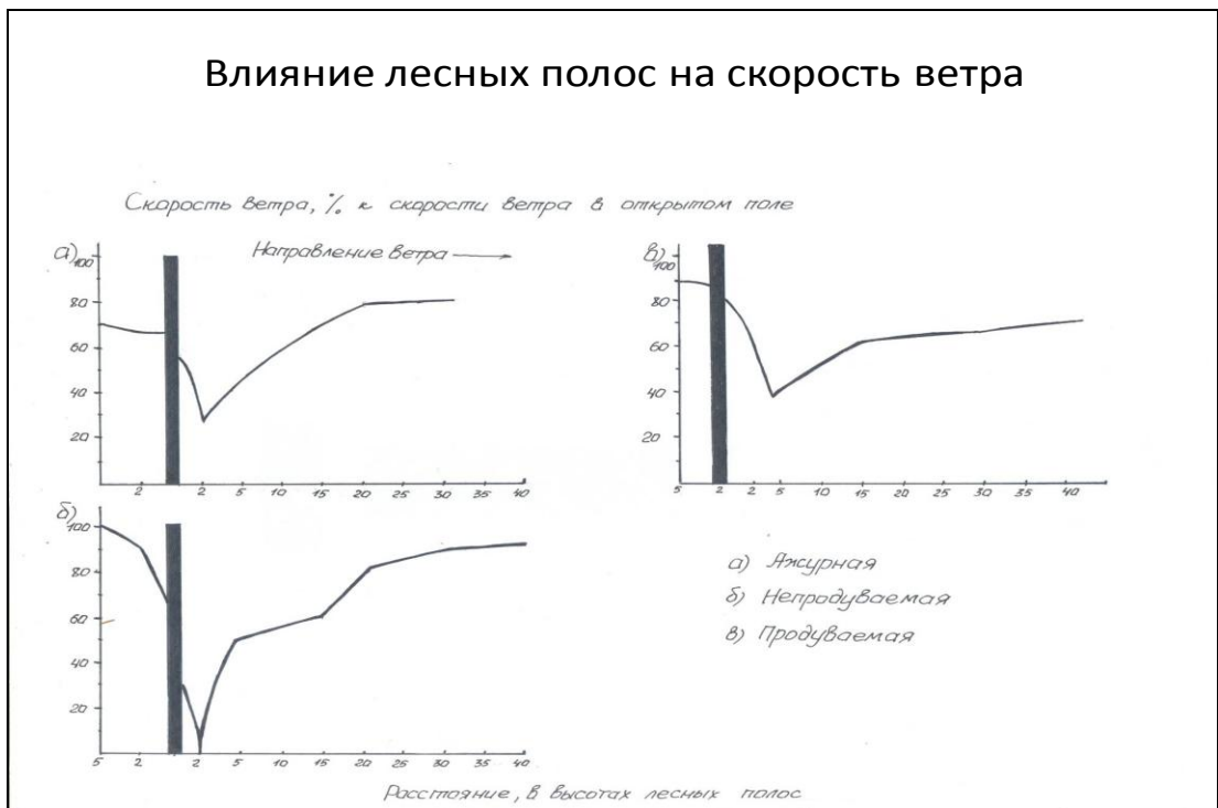
Рисунок 2.2 Влияние лесных полос различной конструкции на скорость ветра
