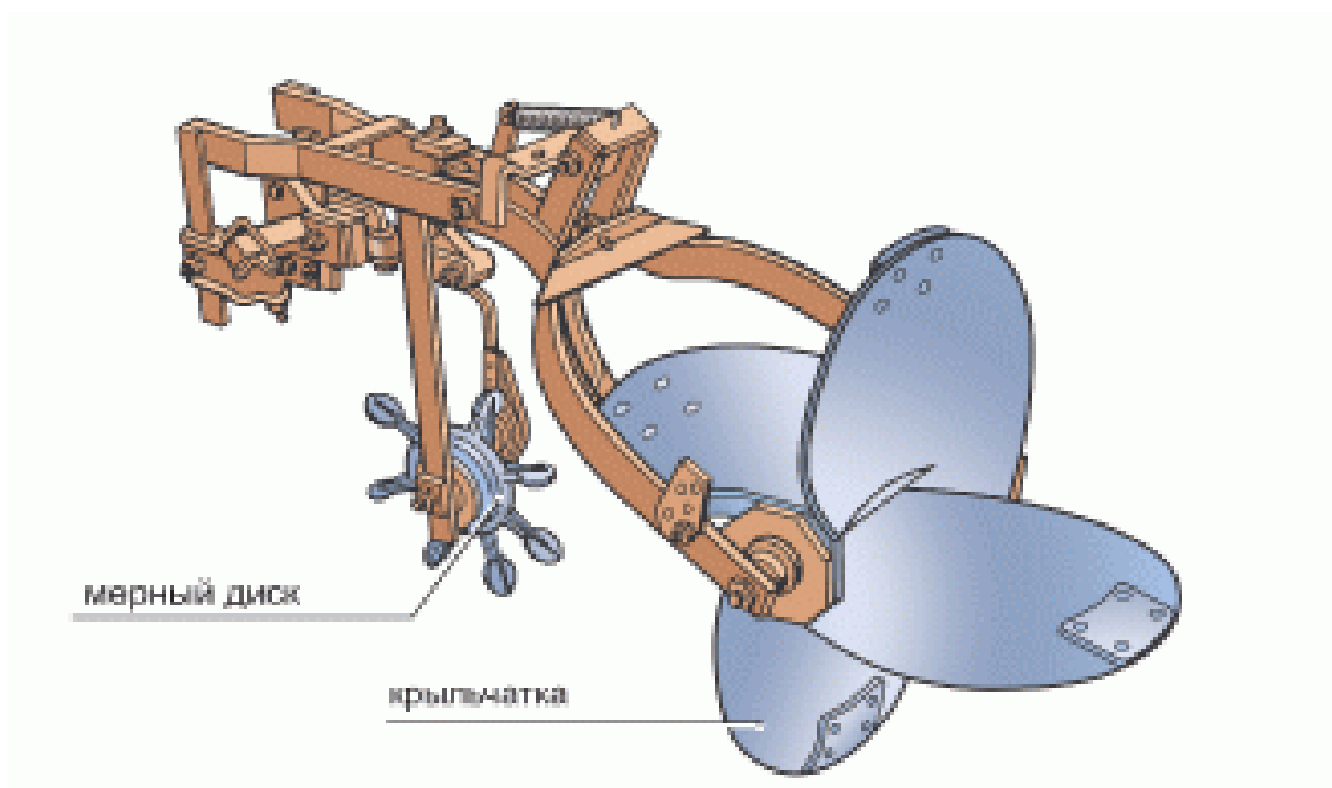
Рисунок 4.10 Лункообразователь ЛОД-10
