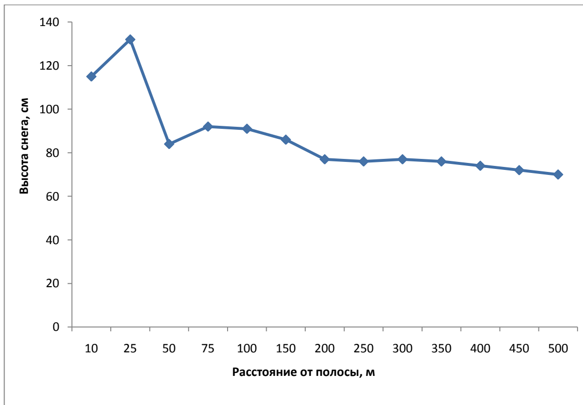
Рисунок 2.4 Профиль снегораспределения на заветренной стороне лесных полос ажурной конструкции
